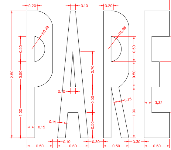
DEMARCACIÓN HORIZONTAL Tipo 10 Total Lámina: 20m
